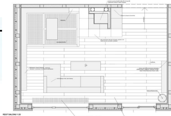
RZUT SALONU 1:25
